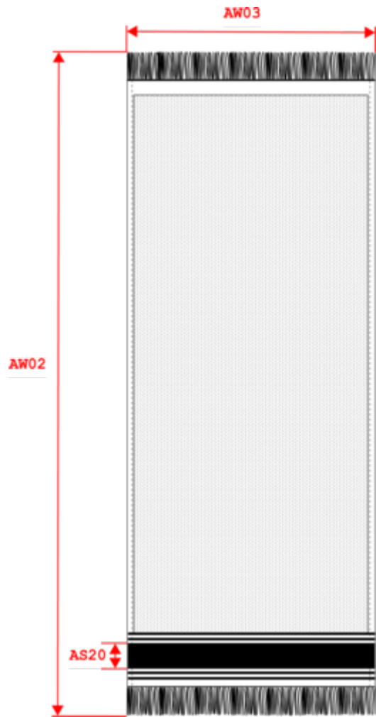
Maße
